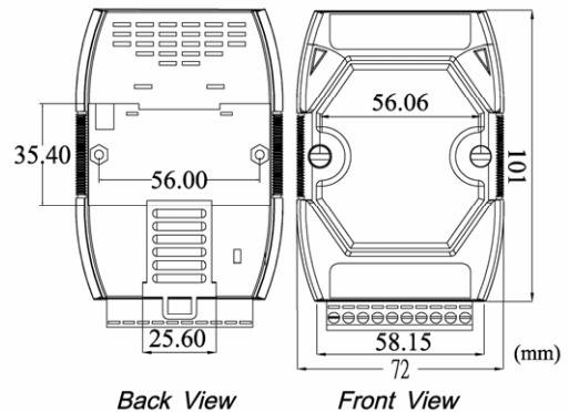
尺寸規格
