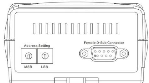
9 針母座 D-Sub 接腳定義
